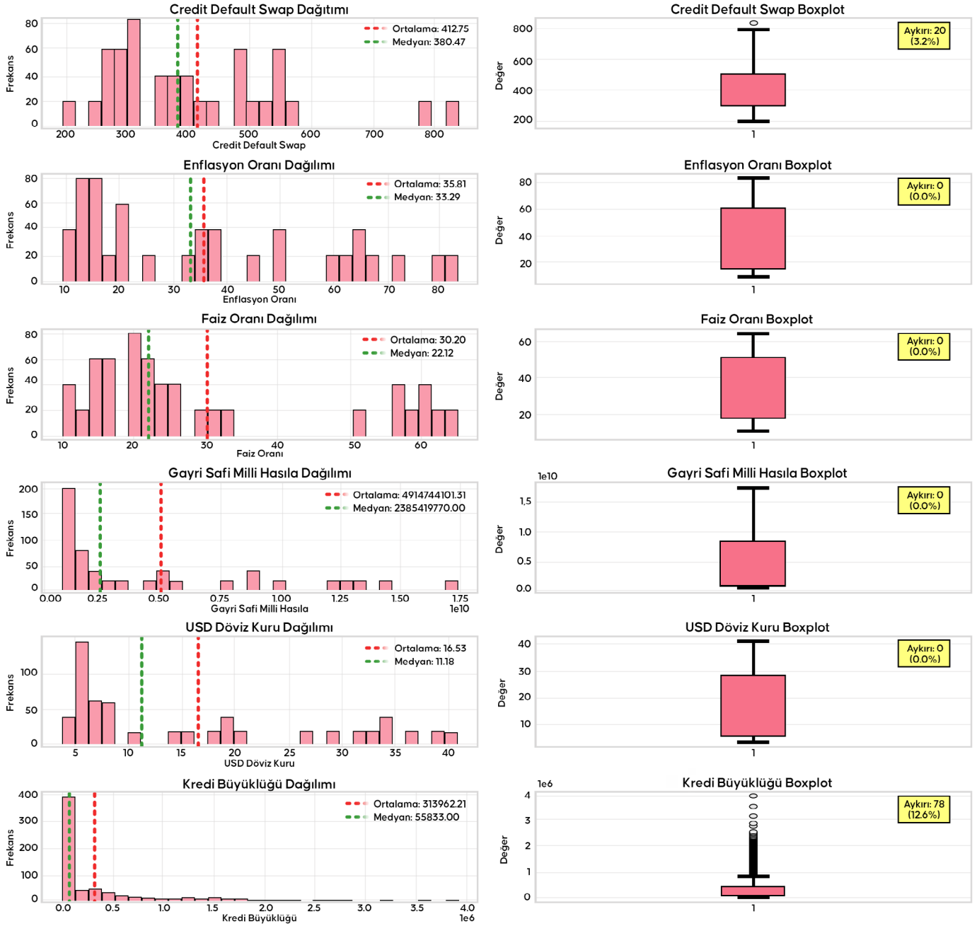
Şekil 1. Değişkenlerin Dağılımı
